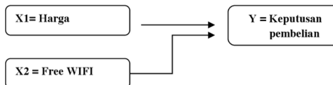
Gambar.1 Kerangka Pemikiran
