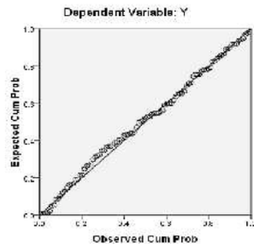
Gambar. 2 Uji Normalitas
